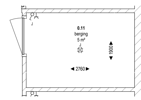
Berging BNR 11 1 : 50
